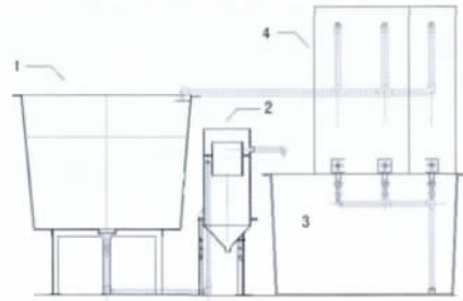
图1 循环水养殖系统示意图
