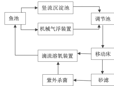
图1 循环水养殖试验系统流程图
